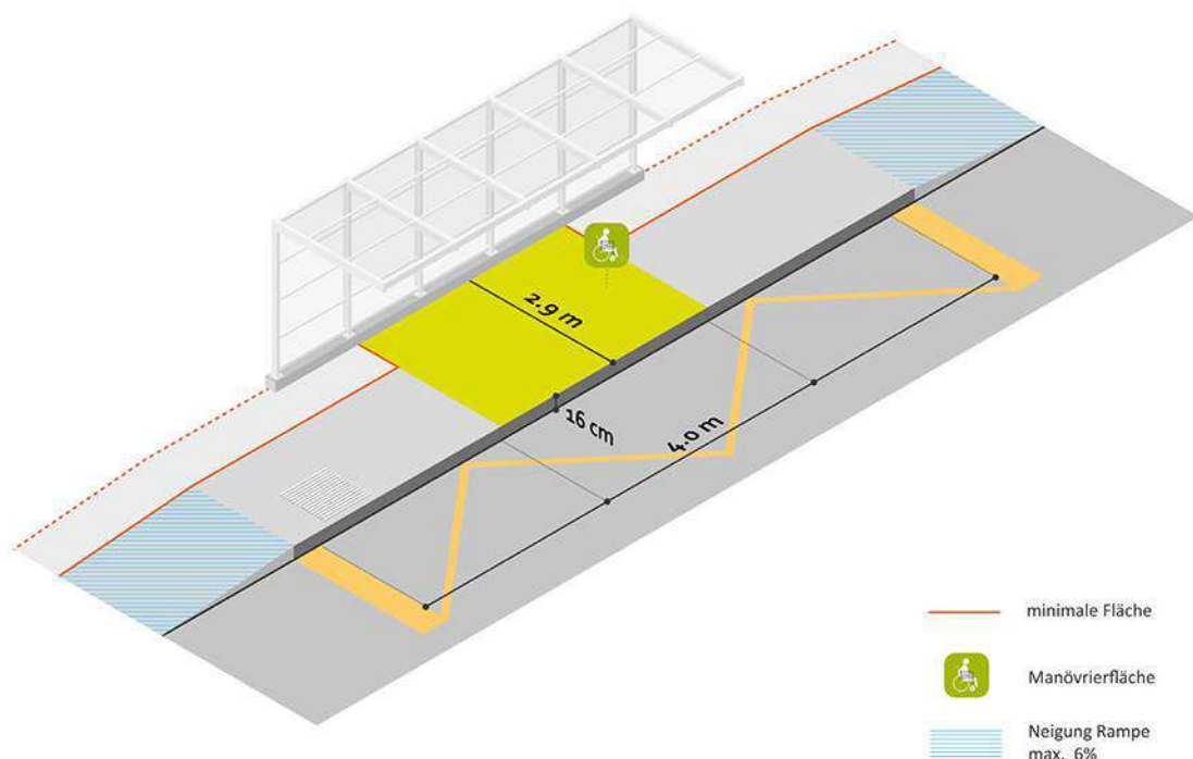
Abbildung 2: Schema Bushaltekante 16 cm
